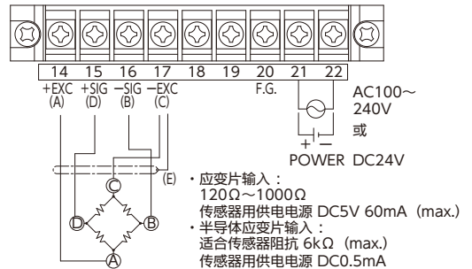
●F4/F5/F6/F8/F9共通 电源、传感器输入用端子台(下段)连接图 过程输入
