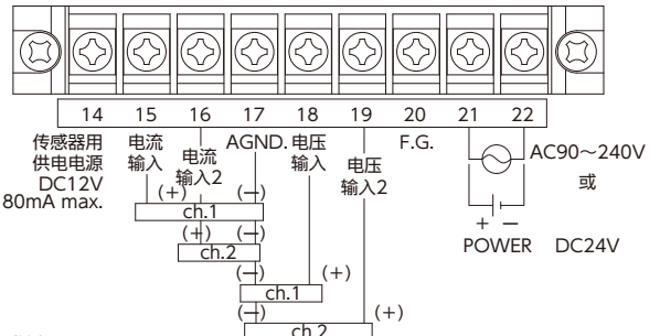
●F4/F5/F6/F8/F9共通 电源、传感器输入用端子台(下段)连接图 过程输入
