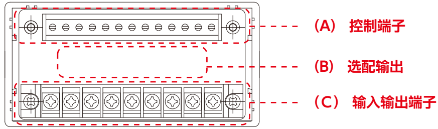
(A) 控制端子连接图 ●F3/F4/F5/F6/F8/F9通用 输出、控制输入用端子台(上段)连接图
