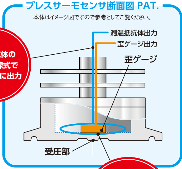
プレスサーモセンサ断面図 PAT.
