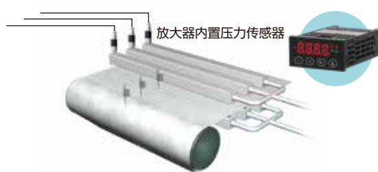
造纸领域抄纸网部分的真空压力监控
