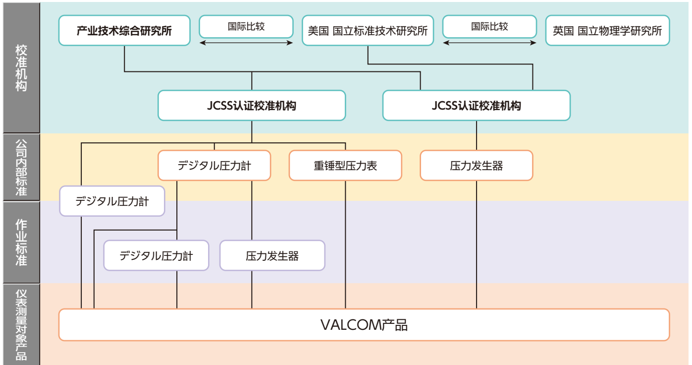
●溯源性体系图（压力）
