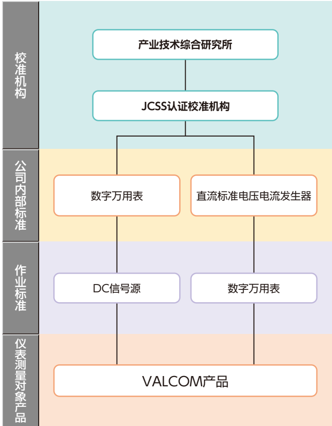
溯源性体系图（电气）
