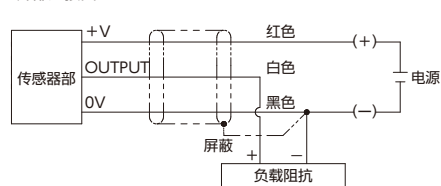
外部连接图
