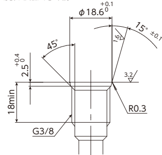
带安装孔传感器尺寸详情
