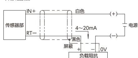
外部连接图
