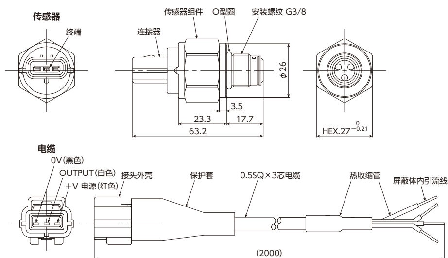
外部连接图
