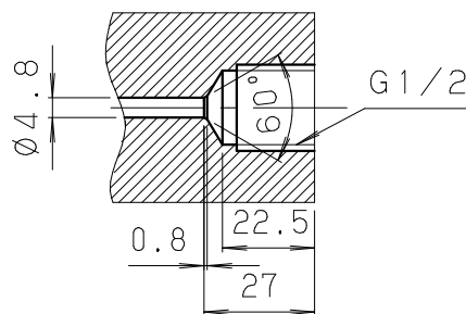
*取付部推奨寸法
