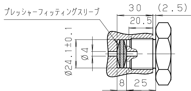
*取付用推奨フィッティング
