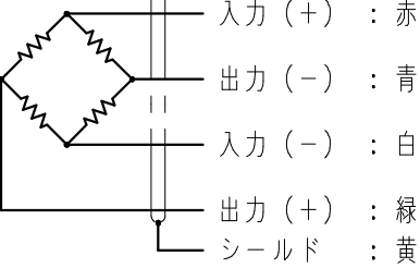
配線図
