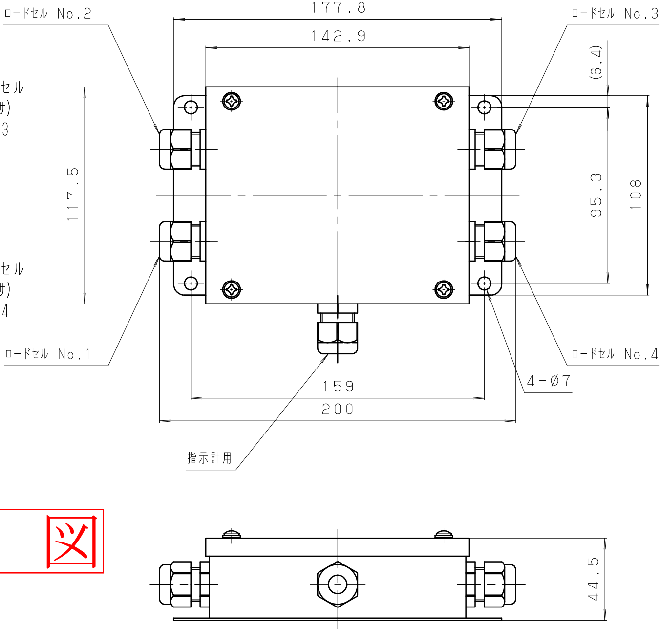
* 外観図
