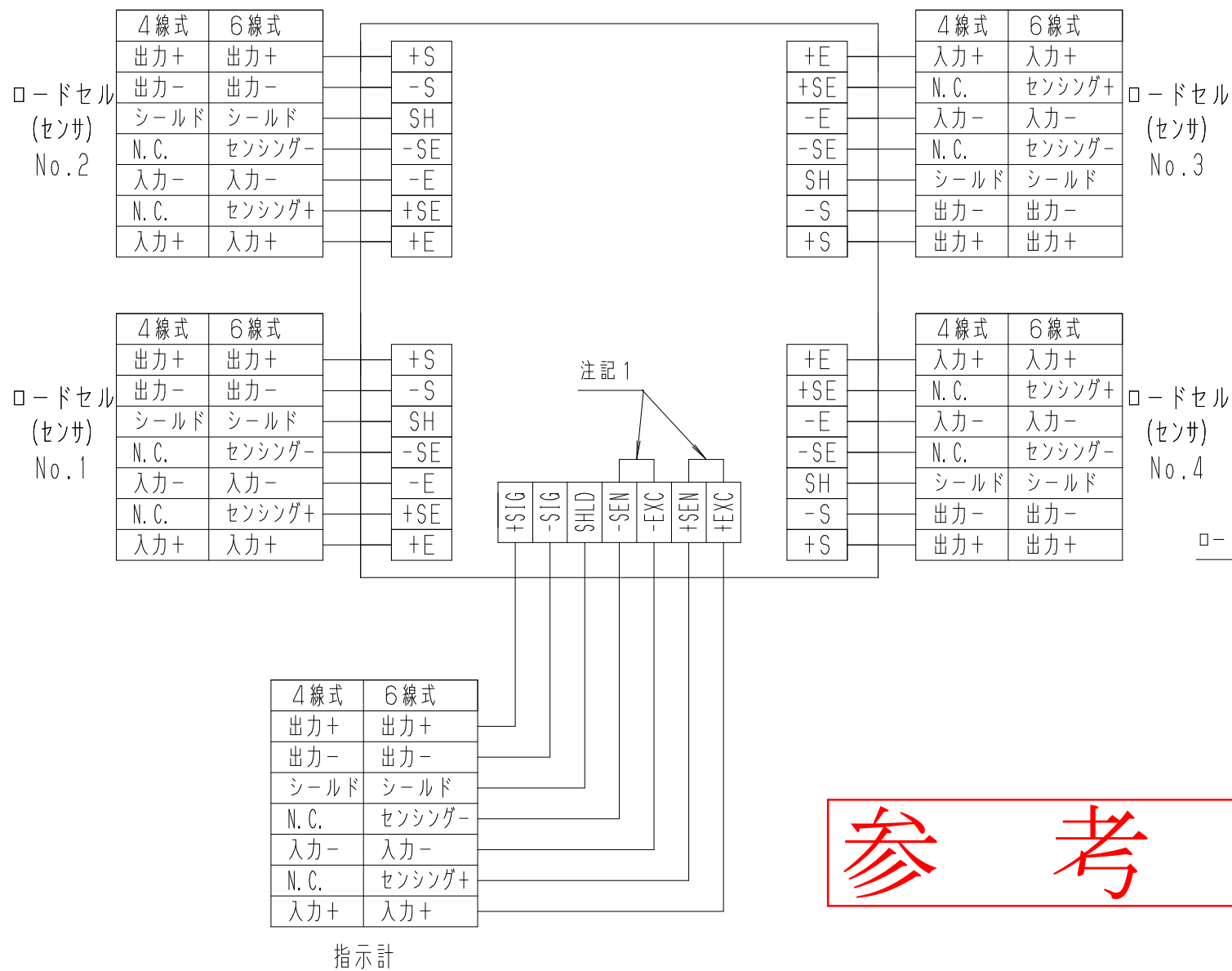
* 配線図
